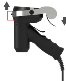
Verstellblech einstellen
